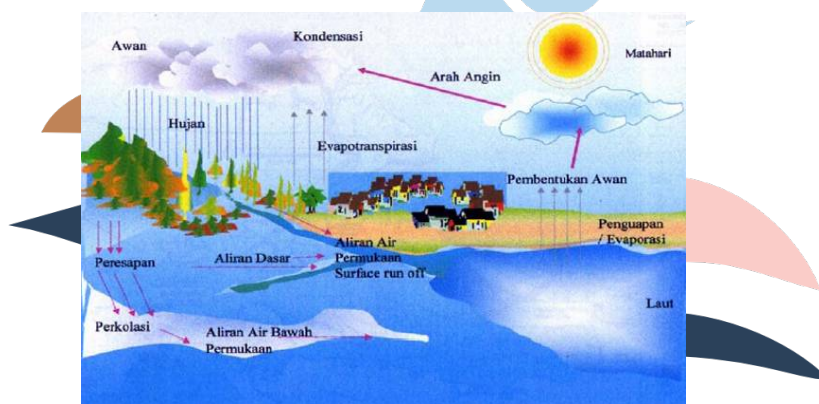
Gambar 2 Daur Air
